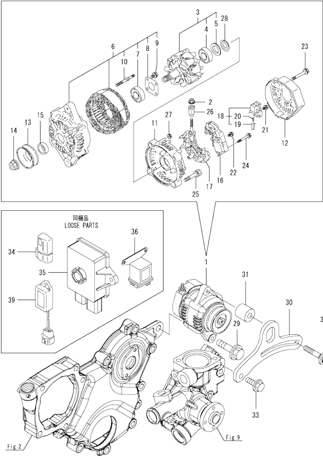
Fig.15. GENERATOR
